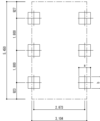
■ 基礎配置図
